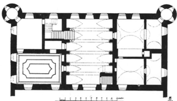
Schloß Ummendorf Grundriß des Erdgeschosses
