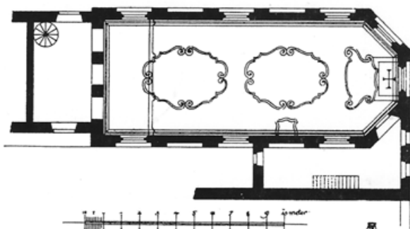
Untersulmetingen Grundriß Kirche
