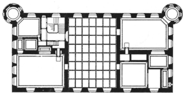
Schloß Ummendorf Grundriß des 2. Obergeschosses
