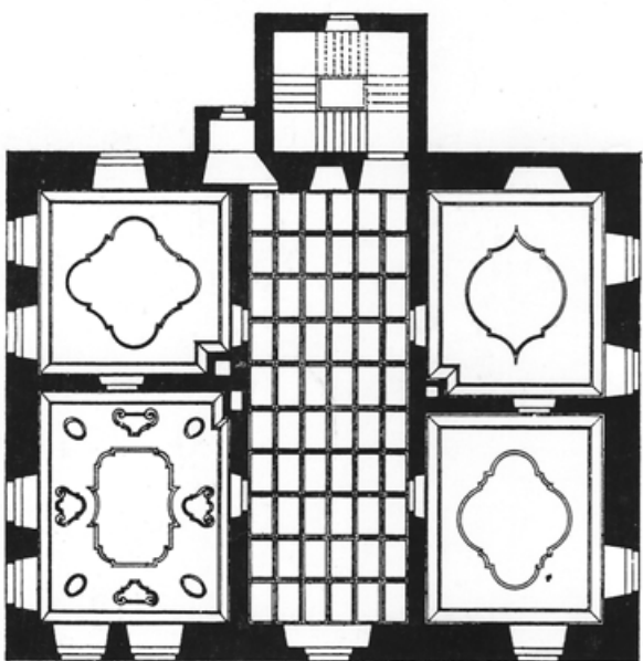
Schloß Untersulmetingen 2. Obergeschloß
